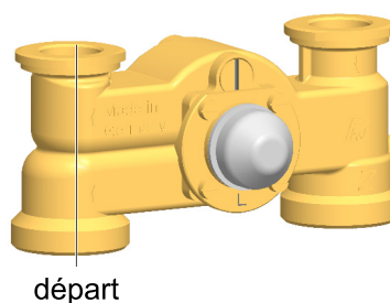
Vanne mélangeuse avec départ à gauche
