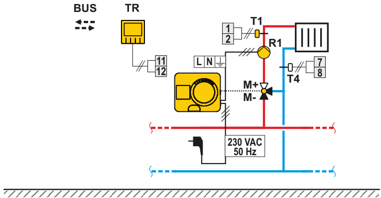
Schéma 360b - circuit de chauffage supplémentaire
