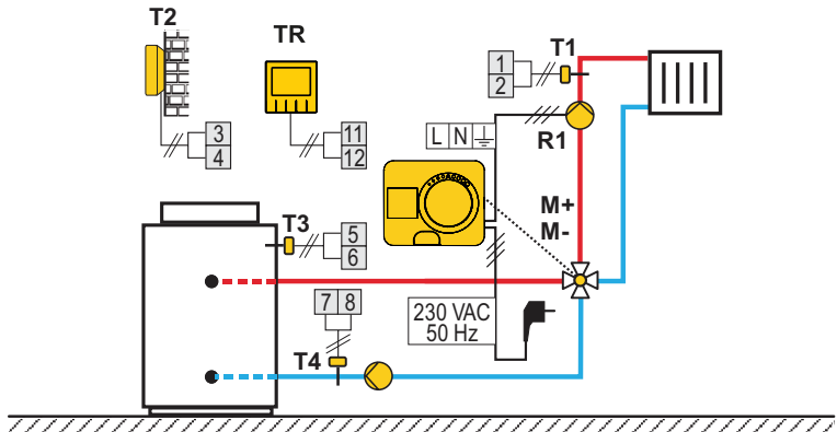
Schéma 361 - Circuit de chauffage et régulation du retour d'eau
